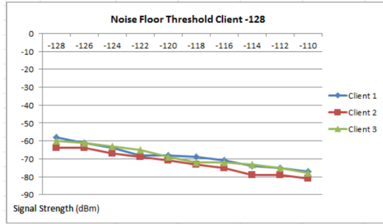
Gambar 5. Grafik Hasil Pengujian Access Point ke 3 Client
