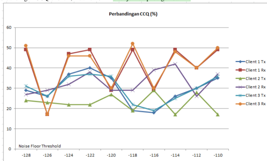
Gambar 11. Grafik Perbandingan CCQ client 1, 2 dan 3 ke AP
