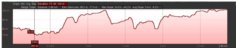
Gambar 2. Kondisi kontur tanah Access Point dan Client 1
