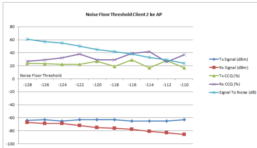
Gambar 8. Grafik Pengujian Signal Strength client 2 ke AP
