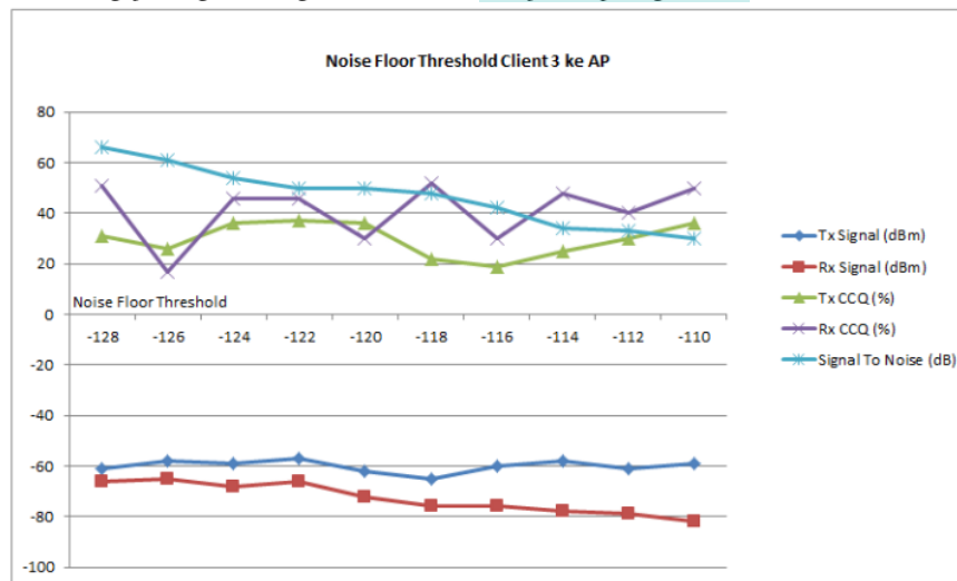
Gambar 9. Grafik Pengujian Signal Strength client 3 ke AP
